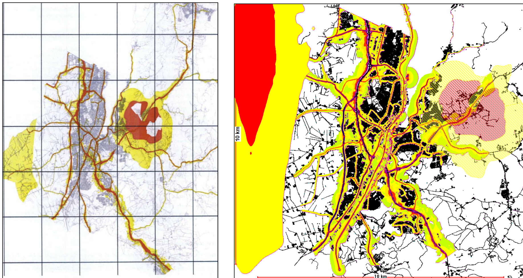
Figur 1 Samlet støysonekart fra hhv. 2012(til venstre) og 2017 (til høyre)
