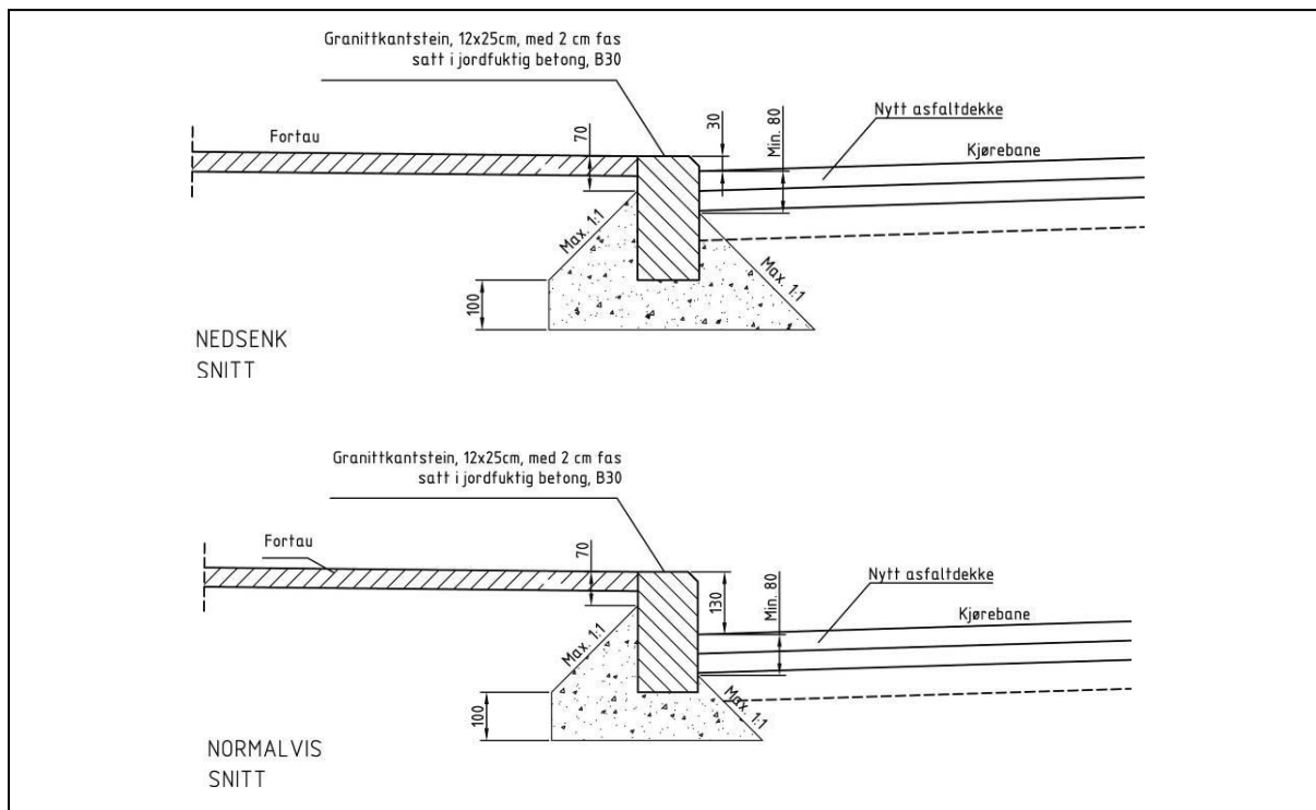
Detalj smal kantstein (Ikke i målestokk. Alle mål i mm)
